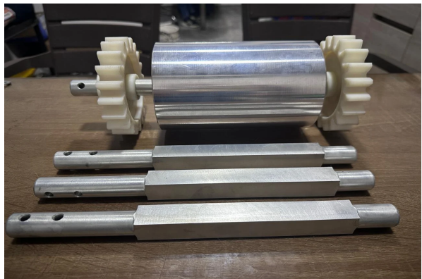
Conjunto de rodillo y engranajes
